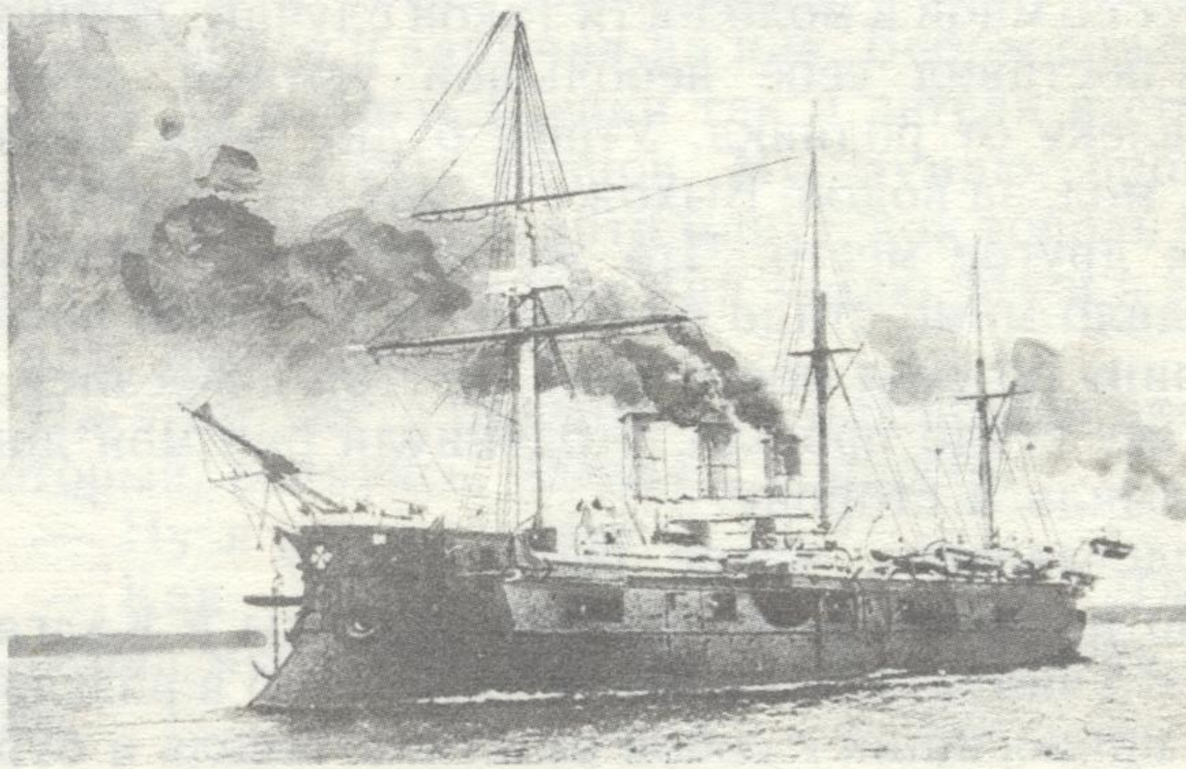
Крейсер I ранга «Память Азова»
